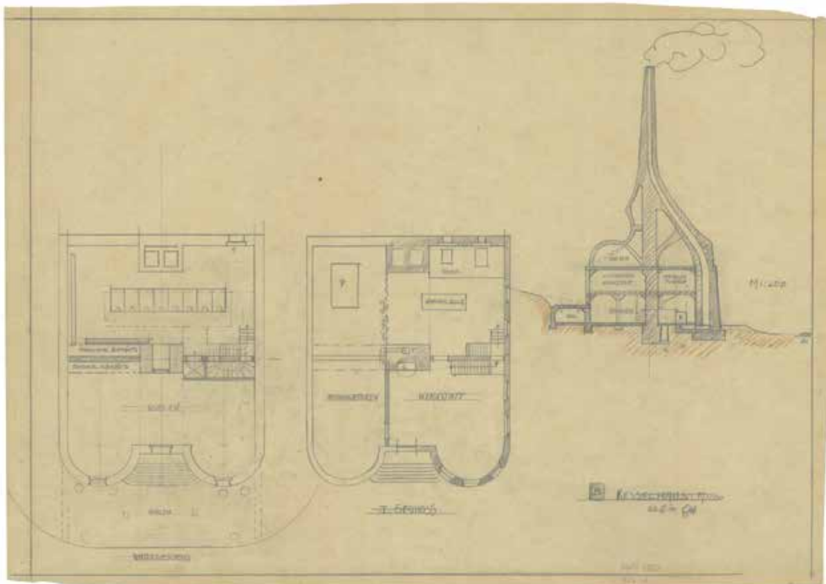
Carl Schmid-Curtius, Grundrisse und Längsschnitt des Heizhauses für den Johannesbau, 1914
