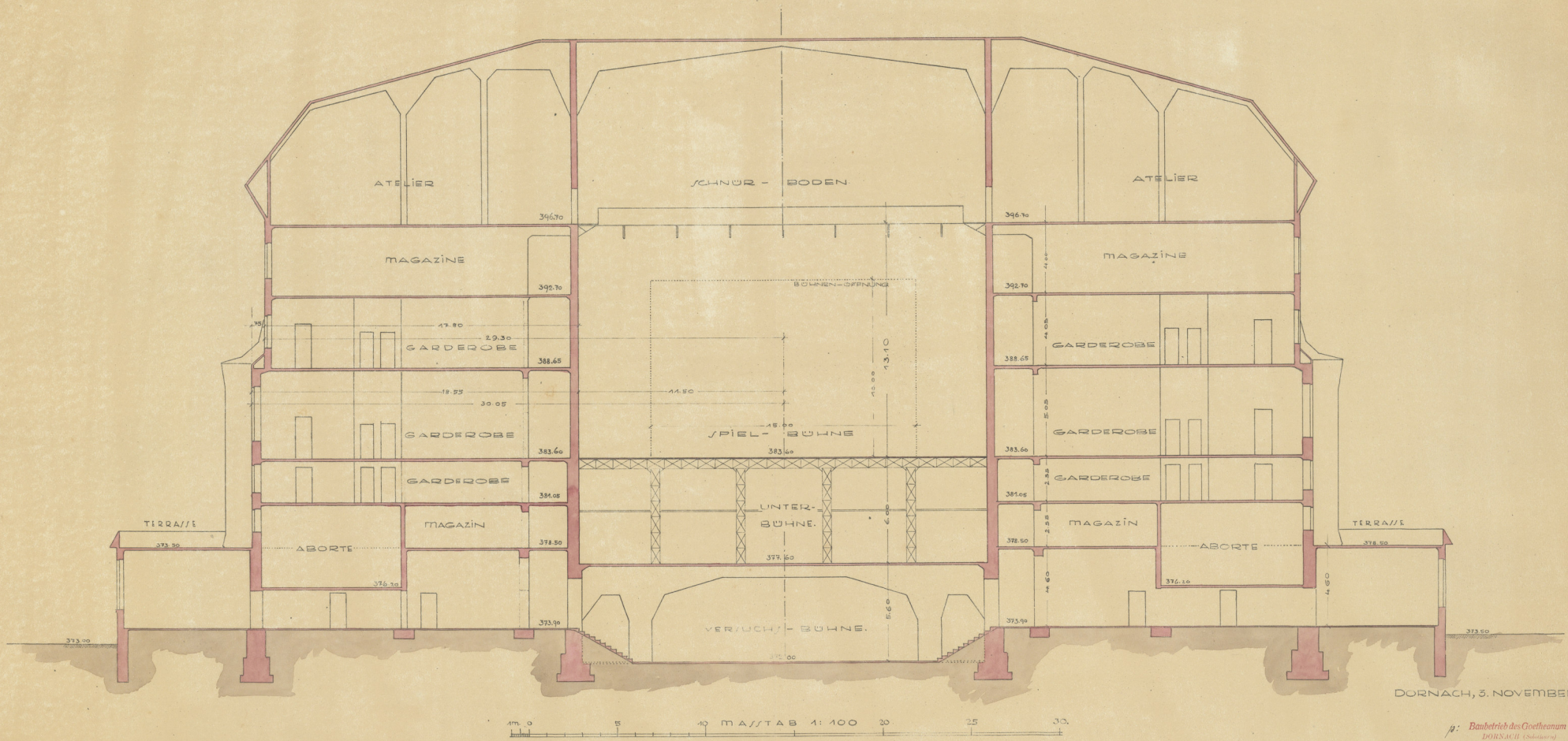
GOETHEANUM QUERSCHNITT A-B DURCH DIE SEITENFLÜGEL.
