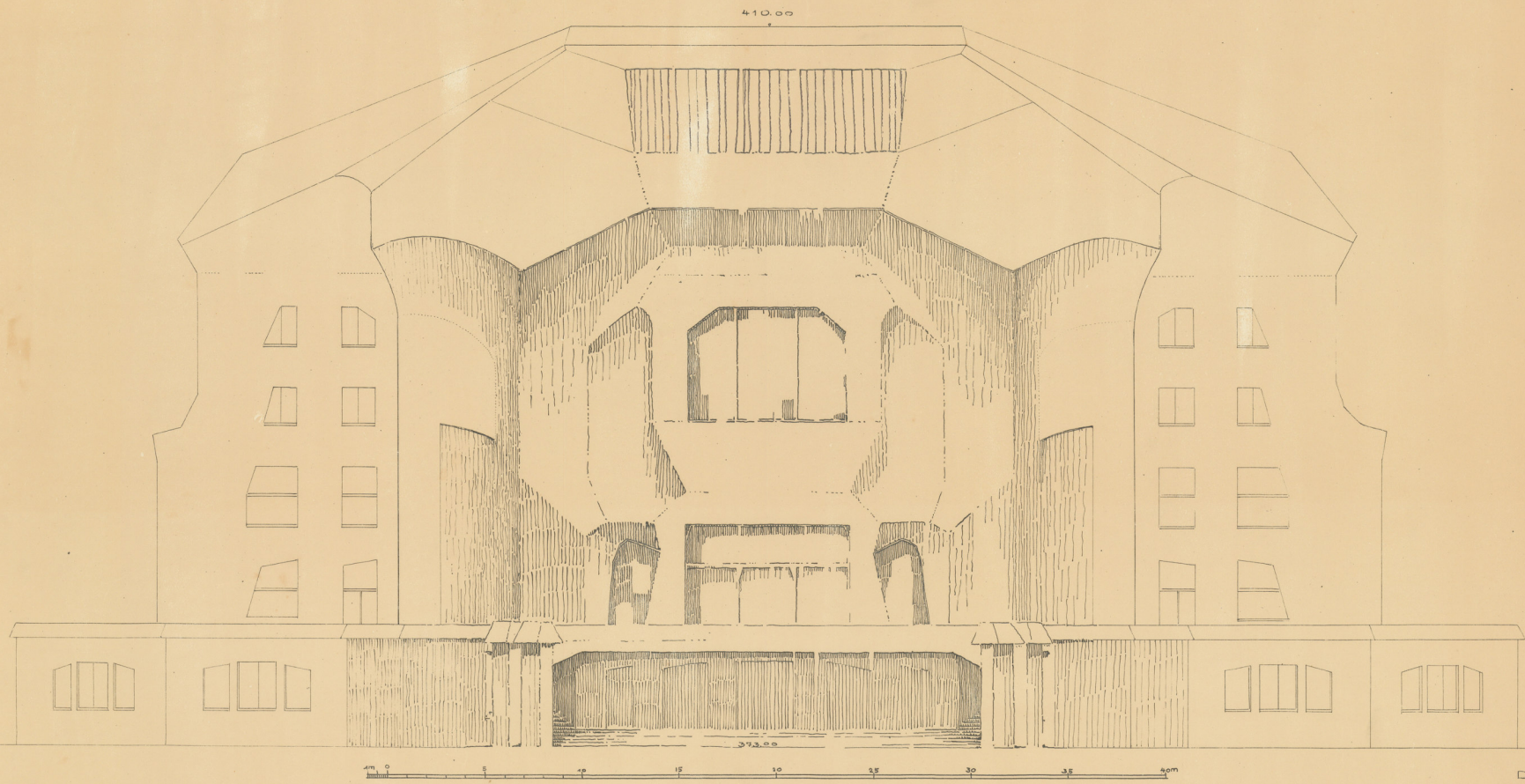
GOETHEANUM WEST-SEITE MASS: 1:100.
