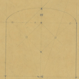
BOGEN ZWISCHEN DEN SÄULENFÜNDAM. 1/2 FELD I. D. AXE. INNERE ANSICHT
