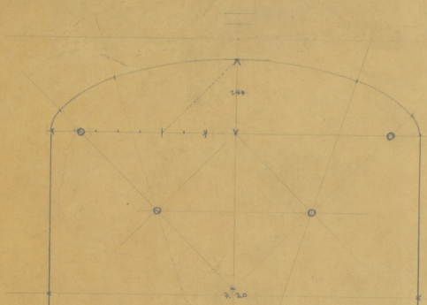
BOGEN VOM UMGANG ZUR GÄRDEROBE (1/2 FELD IN DER AXE) ÄUSSERE ANSICHT
