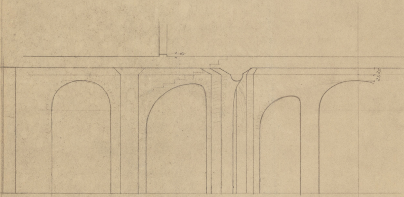
SCHNITT A-D.
