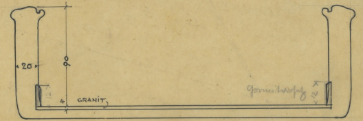
QUERSCHNITT DURCH DIE TREPPE.
