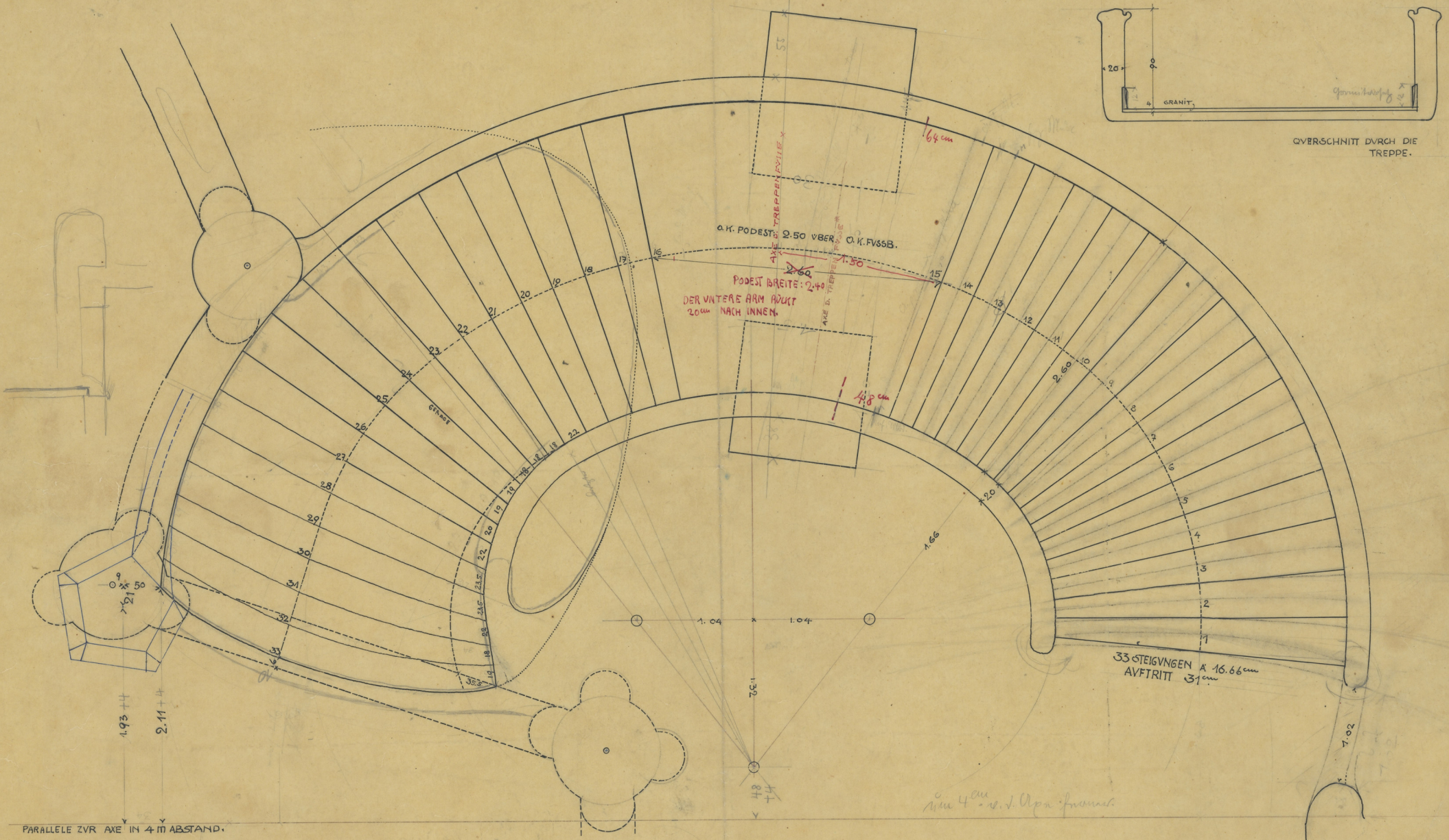
HAVPTTREPPE IM WESTL. VORBAV. M. I/20.
