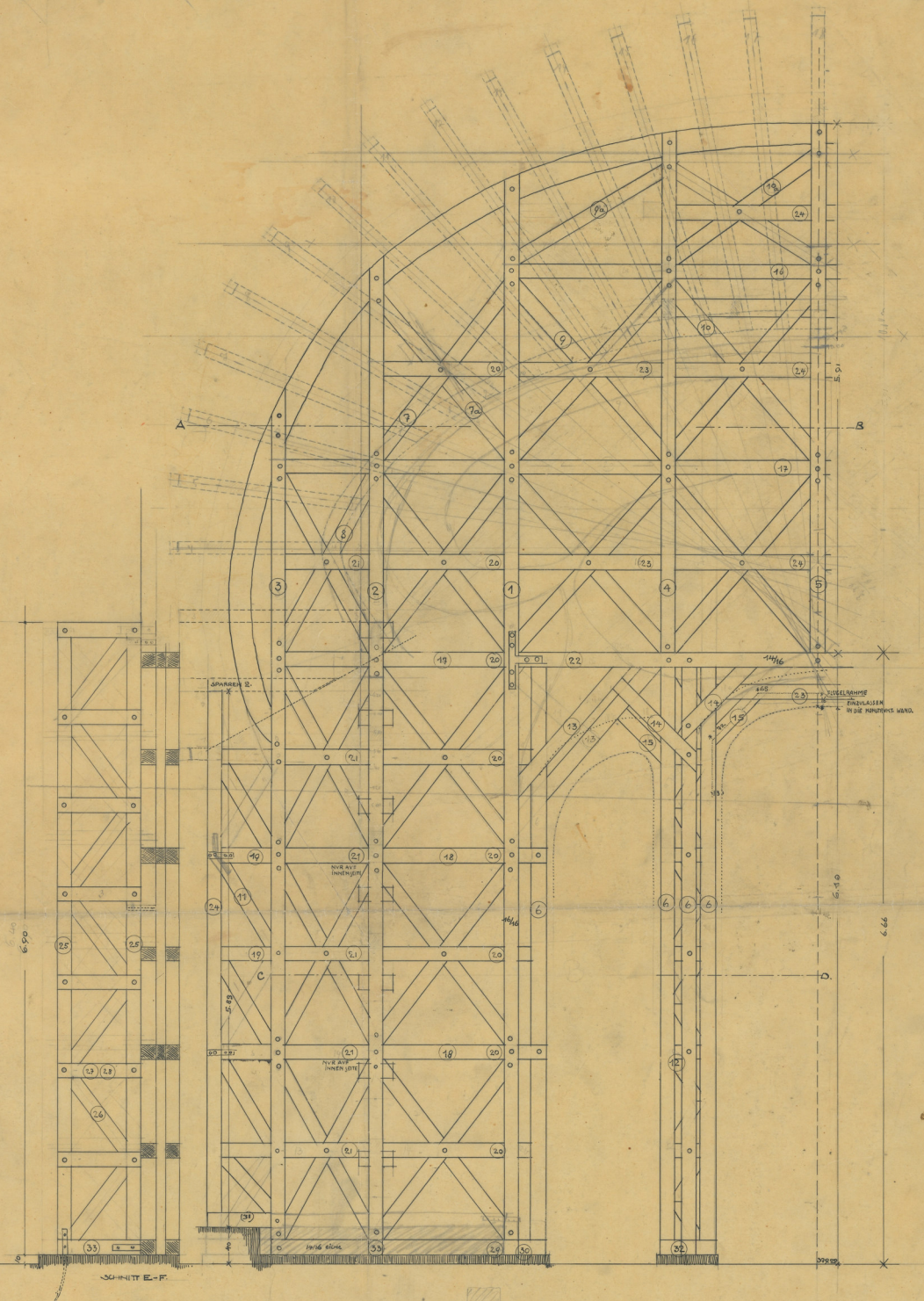
JOHANNESBAY DORNACH. STIRNWAND DES WESTL. VORBAVES. M. 1/20.
