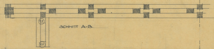
JOHANNESBAY DORNACH. STIRNWAND DES WESTL. VORBAVES. M. 1/20.
