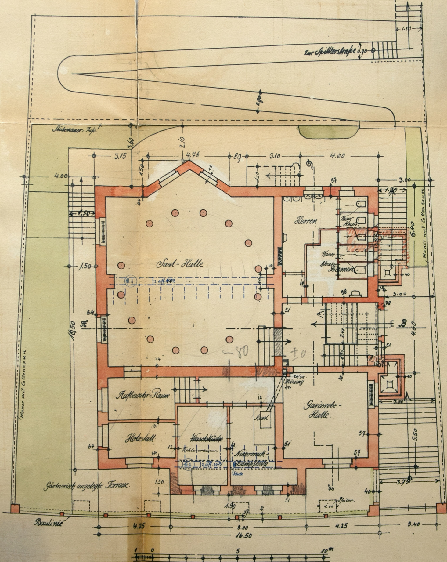
Maßstab 1:100 Erdgeschoss.
